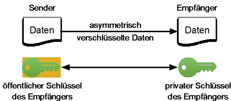
Abbildung 9: Asymmetrische Verschlüsselung
