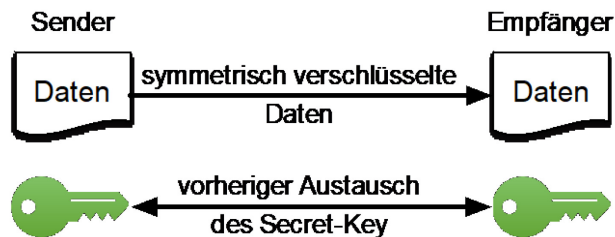
Abbildung 8: Symmetrische Verschlüsselung
